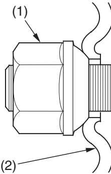
(2) wheel rim
